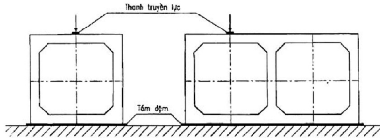
Hình 4 - Vị trí đặt lực để kiểm tra khả năng chịu tải của đốt cống
