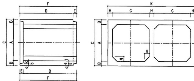
Hình 2 - Đốt cống đôi
