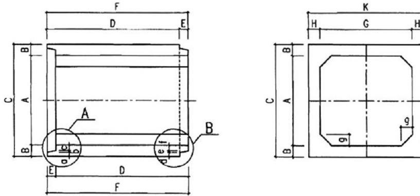
Hình 1 - Đốt cống đơn
